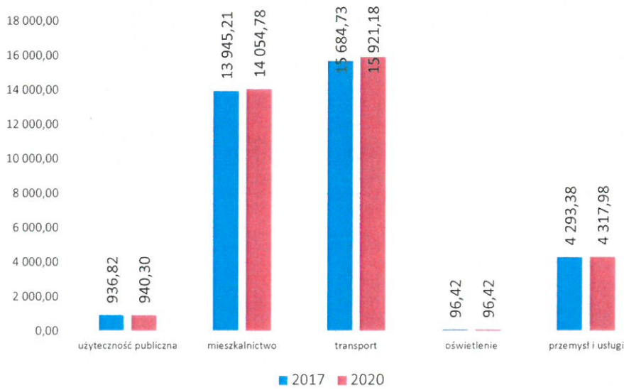
Wykres 22 Prognoza emisji CO 2 w gminie Debrzno w podziale na sektory
