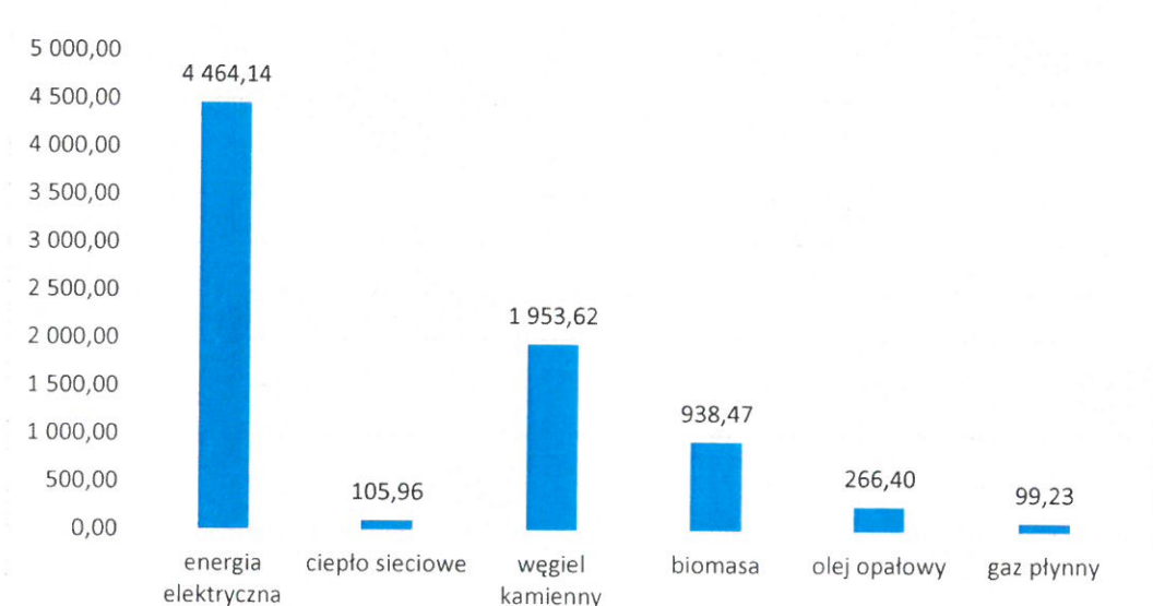
Wykres 12 Zużycie energii w sektorze przemysłu i usług
