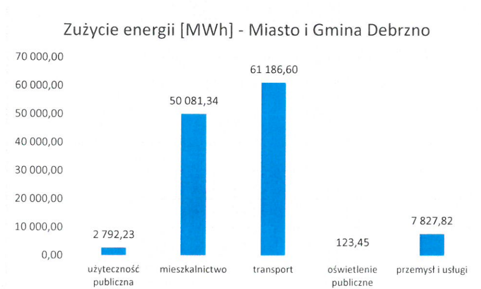
Wykres 15 Zużycie energii w gminie Debrzno w podziale na sektory
