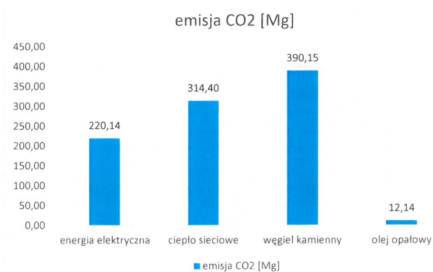
Wykres 3 Emisja CO 2 w budynkach użyteczności publicznej
