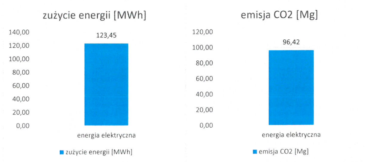
Wykres 11 Zużycie energii oraz emisja CO 2 związana z oświetleniem gminnym
