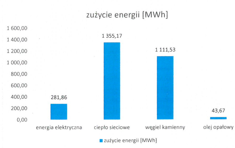
Wykres 2 Zużycie energii w budynkach użyteczności publicznej
