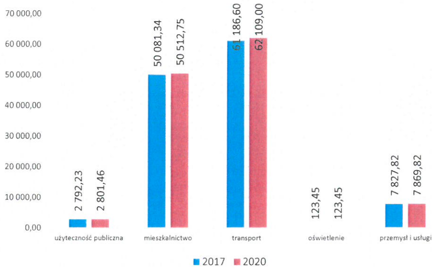
Wykres 21 Prognoza zużycia energii w gminie Debrzno w podziale na sektory
