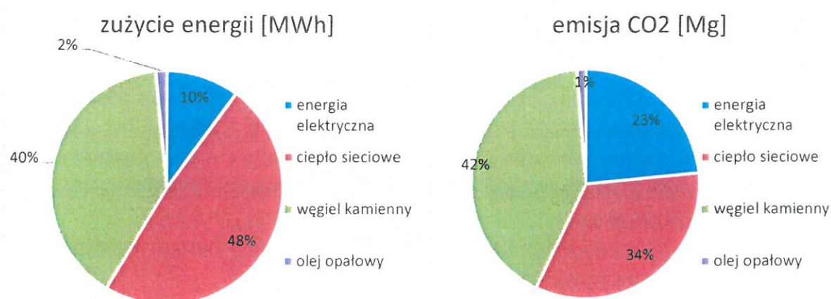
Wykres 4 Udział nośników energii w budynkach użyteczności publicznej
