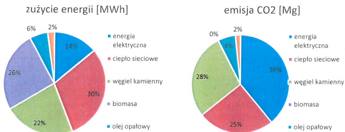
Wykres 7 Udział nośników energii w sektorze mieszkalnictwa
