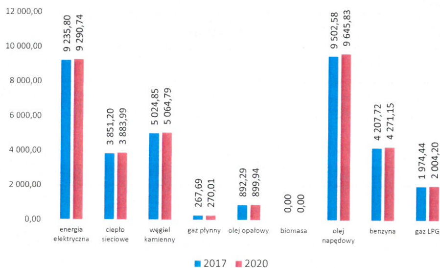
Wykres 24 Prognoza emisji CO 2 w gminie Debrzno w podziale na nośniki energii
