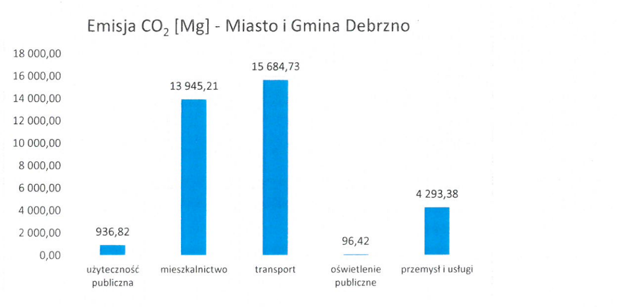
Wykres 16 Emisja CO 2 w gminie Debrzno w podziale na sektory
