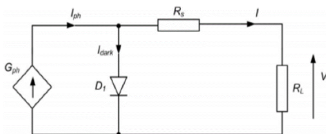
Rysunek 5 Schemat elektryczny ogniwka
